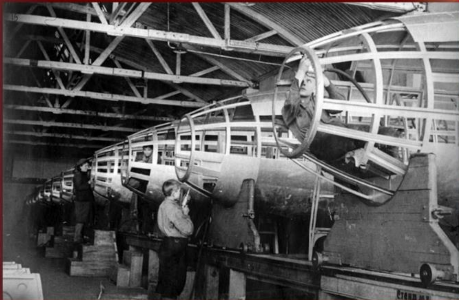
Цех завода Хабаровского авиационного завода № 83 им. М. Горького. г. Хабаровск. 1940-е гг. Из фондов музея истории г. Хабаровска
